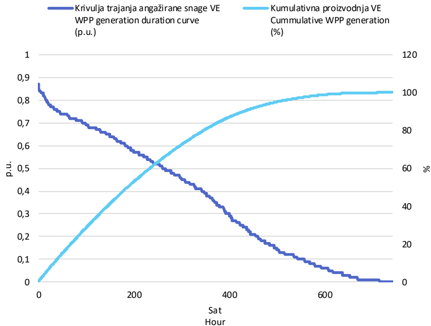
Slika 3 Krivulja trajanja angažirane snage svih VE i kumulativna proizvodnja VE u ožujku 2025. godine u jediničnim vrijednostima
