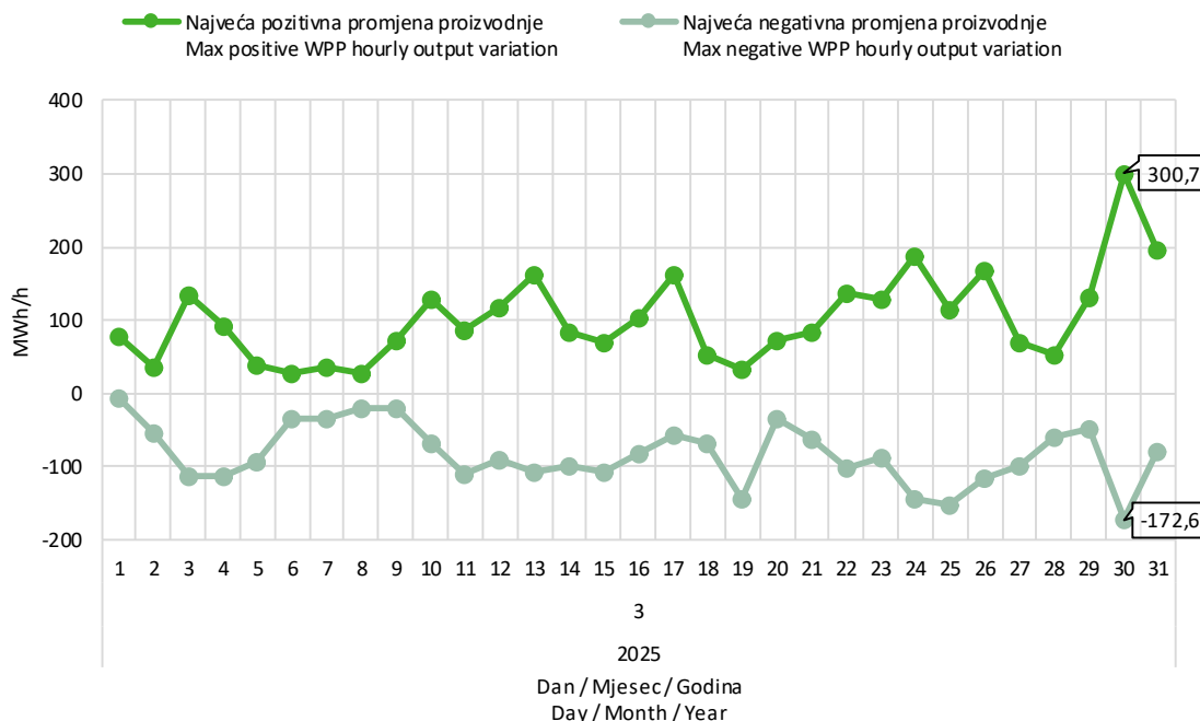
Slika 9 Maksimalna pozitivna i maksimalna negativna promjena satne proizvodnje VE u ožujku 2025. godine
