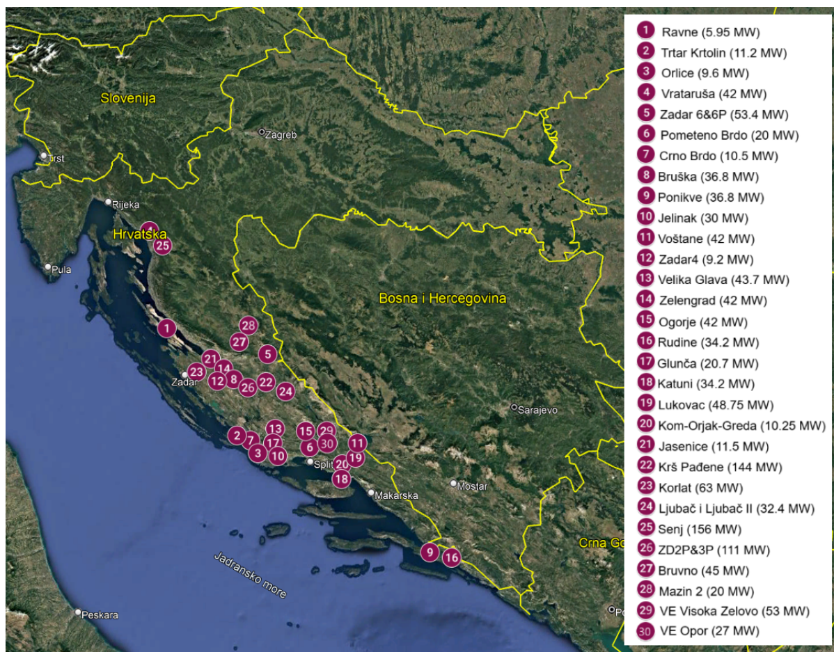
Slika 1 Lokacije VE u Hrvatskoj
