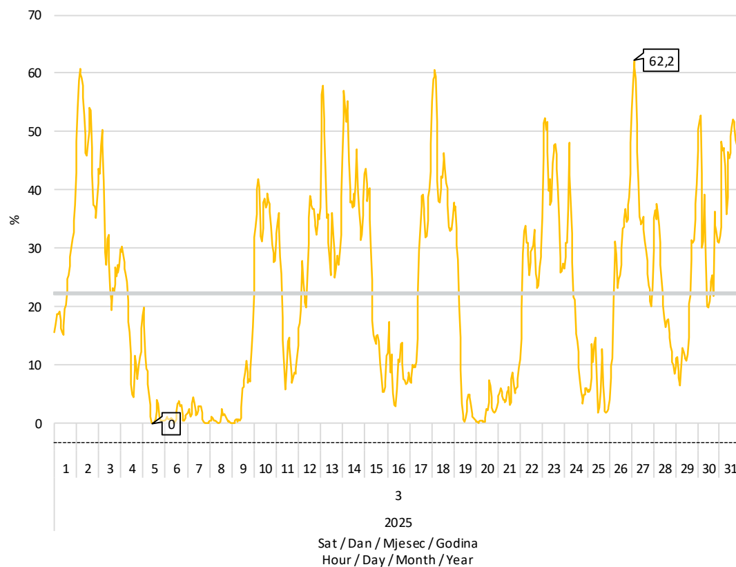
Slika 8 Udio proizvodnje vjetroelektrana u pokrivanju satnog opterećenja elektroenergetskog sustava u ožujku 2025. godine
