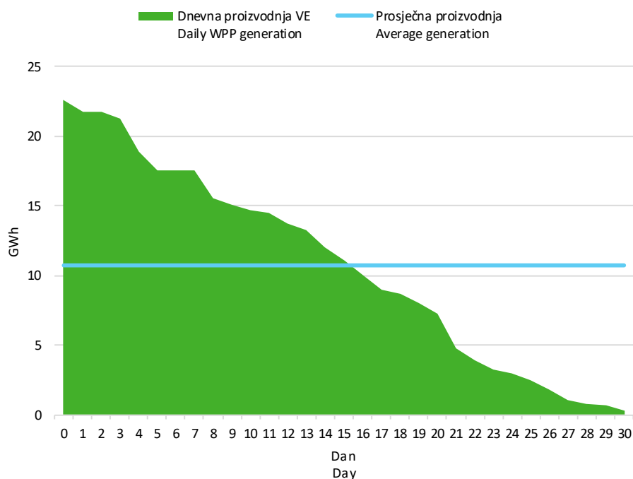
Slika 6 Krivulja trajanja dnevne proizvodnje vjetroelektrana u ožujku 2025. godine
