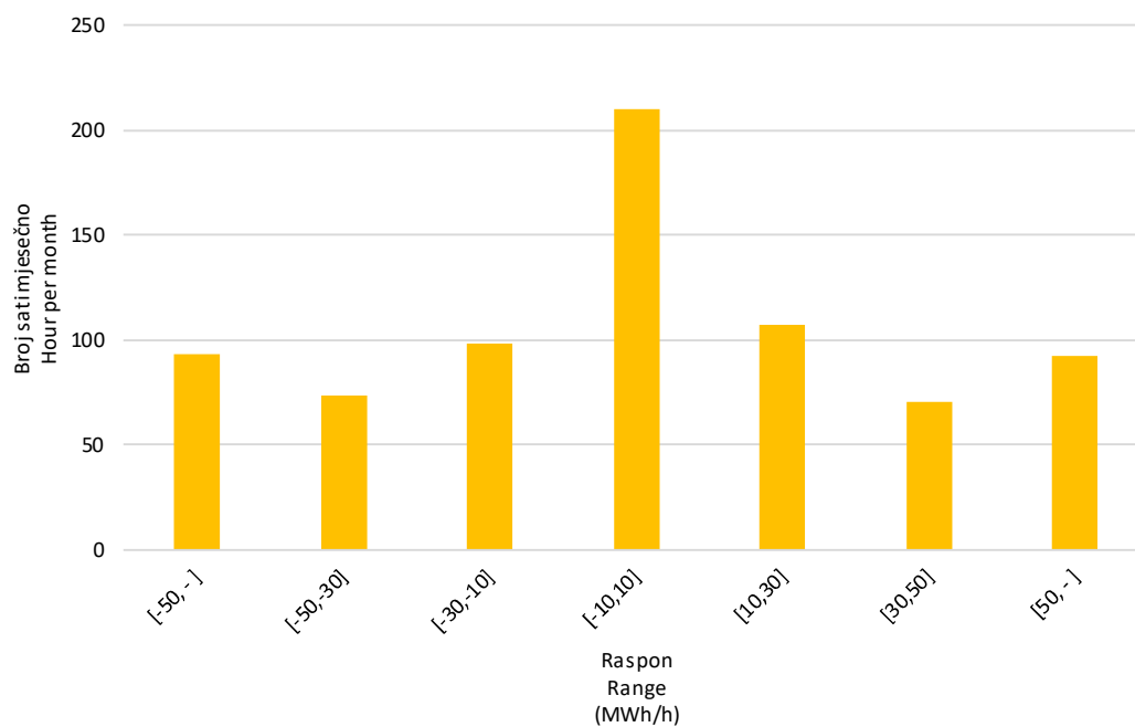
Slika 10 Statistička raspodjela satnih promjena proizvodnje VE u ožujku 2025. godine
