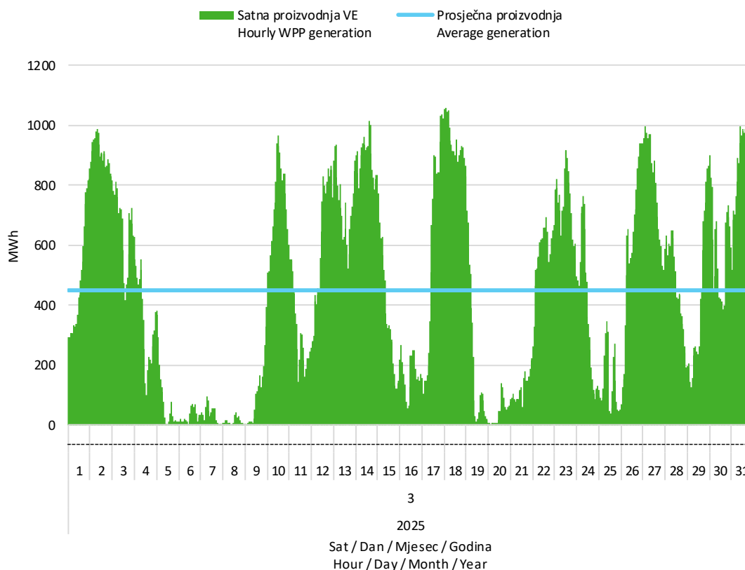
Slika 2 Satna proizvodnja svih vjetroelektrana u ožujku 2025. godine
