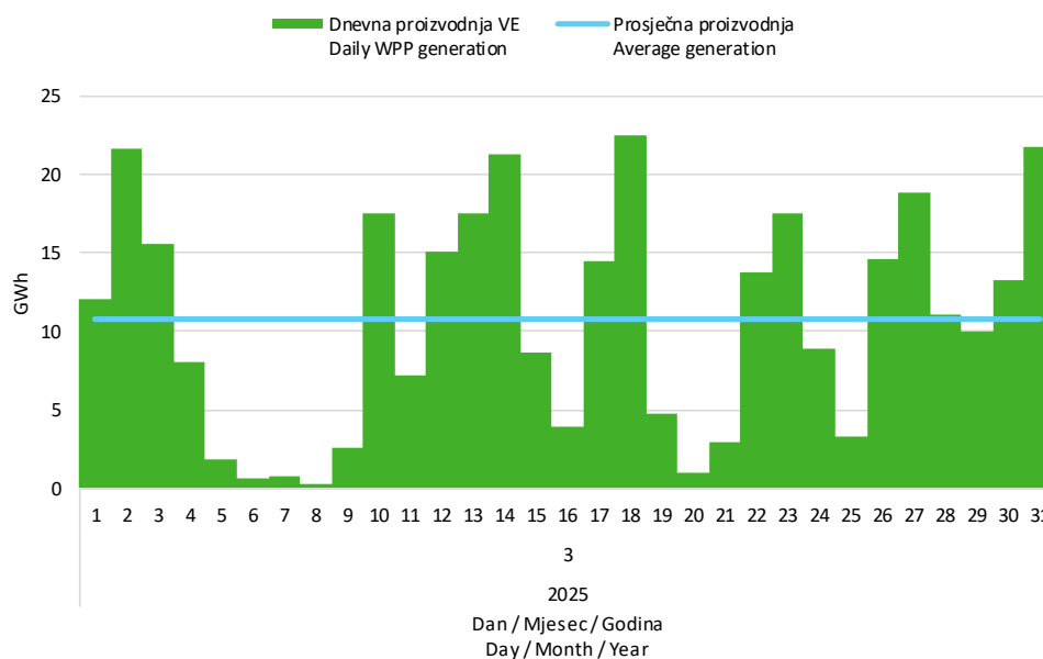
Slika 5 Dnevna proizvodnja svih vjetroelektrana u ožujku 2025. godine
