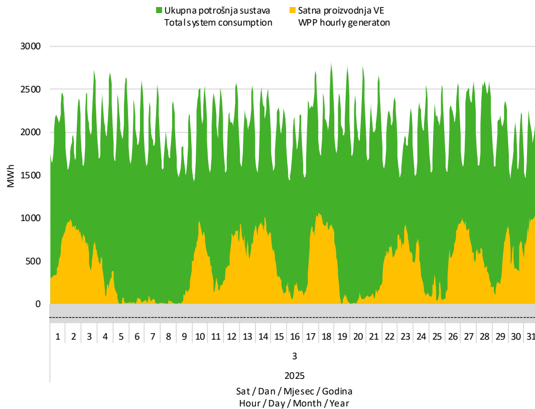
Slika 7 Usporedba satnog dijagrama opterećenja sustava i proizvodnje vjetroelektrana u ožujku 2025. godine
